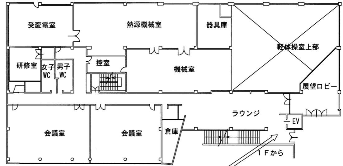
2F 平面図
